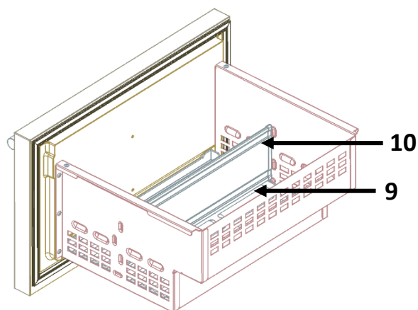
Tiroir inférieur
