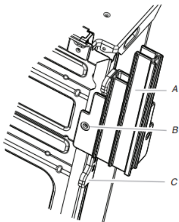
A. Pied avant B. Vis no 8-18 x 3/8 po (9,5 mm) C. Cale
