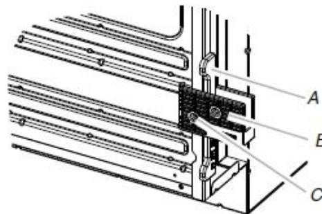
A. Cale B. Pied arrière C. Vis no 8-18 x 3/8 po (9,5 mm)
