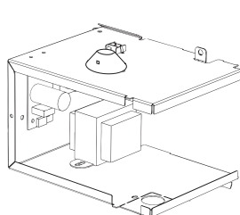
Boîte de jonction
