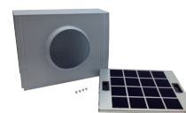
HCREC5UC Recirculation kit
