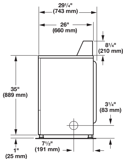
Vista lateral
