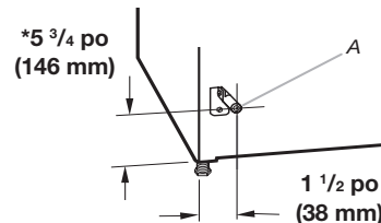
A. Conduit NPT de la sècheuse de 3/8 po
