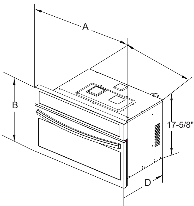
Figura 2: Sólo microondas
