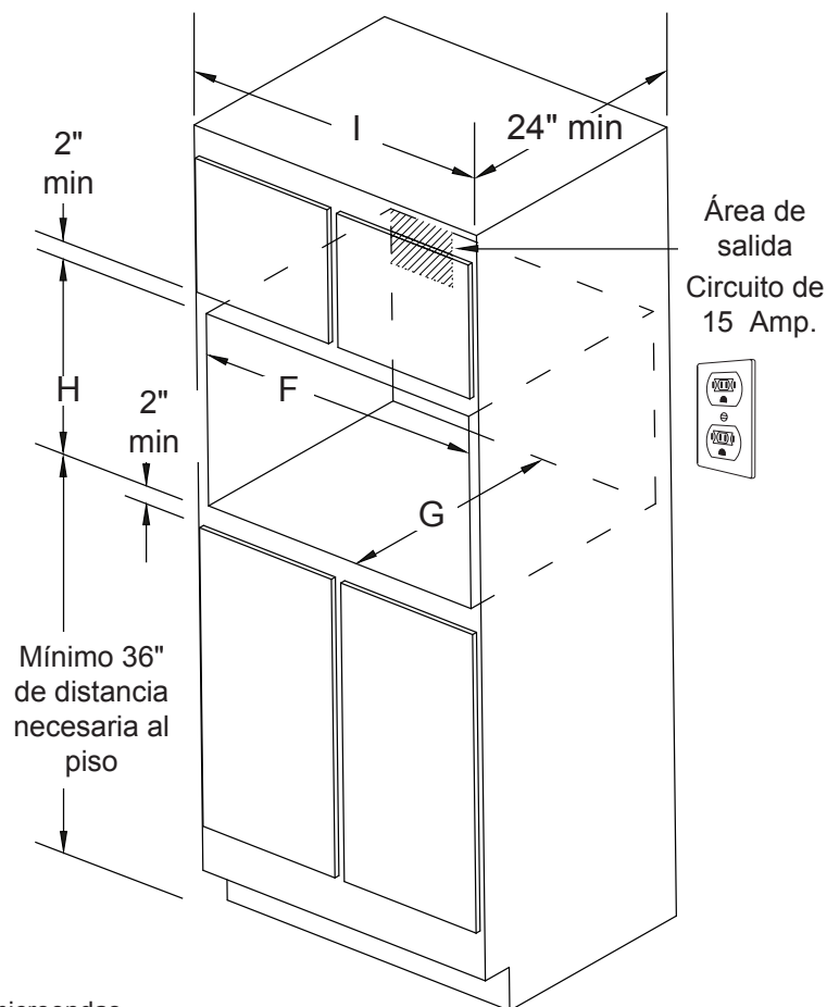
Figura 2: Sólo microondas
