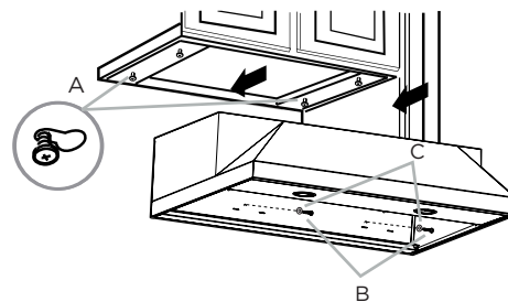
A. 4- Tornillos de montaje B. Tornillos de seguridad C. Rondanas
