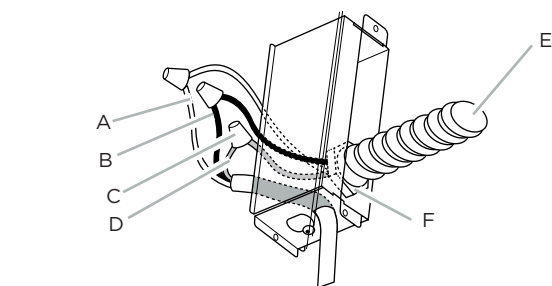
A. Alambres blancos B. Alambres negros C. Conectores de alambres aprobados por UL D. Alambres verdes (o desnudos) y amarillos - verdes de puesta a tierra E. Cable de alimentación F. Sujeta cable de ½" (aprobado por UL o CSA)
