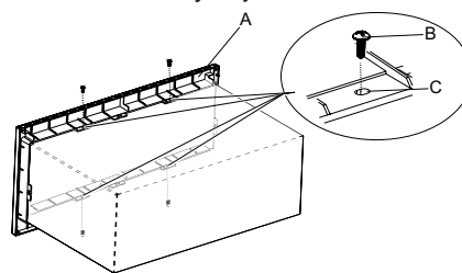
A. Marco del kit de molduras B. Tornillo de cabeza redonda para chapa n.º 7-18 x 7/16" (4) C. Orificio para tornillo (4)
