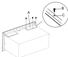
A. Conducto de enfriamiento del lado izquierdo B. Tornillos cortos (3) C. Orificio para tornillo (3)
