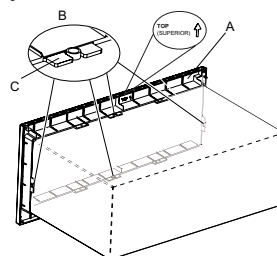
A. Marco del kit de molduras B. Pasador de ubicación (4) C. Ranura de ubicación (4)
