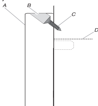
A. Marco del kit de molduras B. Guía del orificio de montaje C. Tornillo de cabeza plana para madera n.º 7-16 x 15/16" (4) D. Parte superior del recorte
