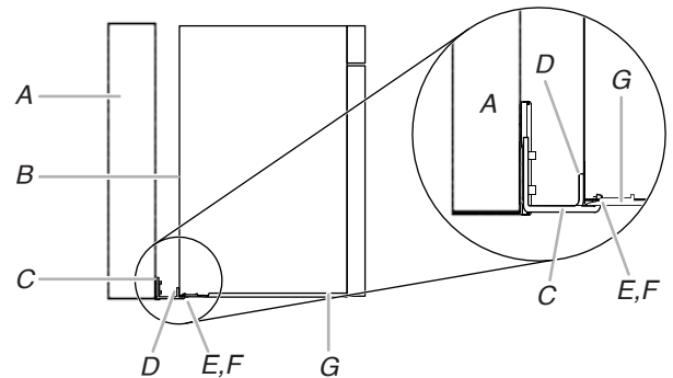
A. Pared B. Parte trasera del horno microondas C. Kit de montaje sobresaliente D. Tope colgante E. Gancho colgante F. Orificio trasero de la placa inferior G. Placa inferior
