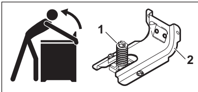
1. Pied de nivellement de la cuisinière / 2. Support anti-basculement
