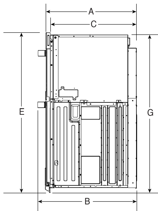
VUE LATÉRALE
