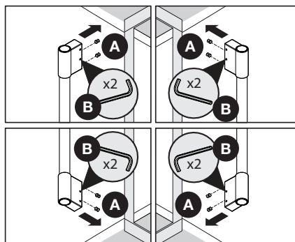
Mounting Refrigerator Handles Montaje de las manijas del refrigerador Assemblage des poignées du réfrigérateur
