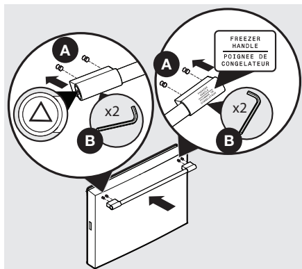
Mounting Freezer Handle Montaje de la manija del congelador Montage de la poignée du congélateur
