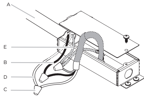
A. Cable de suministro de energía doméstico B. Alambres negros C. Conectores de alambres aprobados por UL D. Alambres blancos E. Alambres verdes (o desnudos) y amarillos - verdes de puesta a tierra
