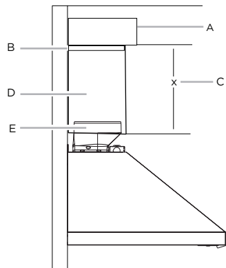
A. Deflector B. Abrazadera para ducto C. X= longitud para cortar el ducto de escape D. Ducto de escape E. Salida de escape
