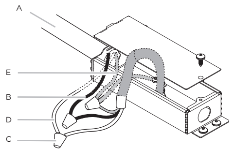
A. Câble d'alimentation électrique du domicile B. Conducteurs noirs C. Connecteurs de fils (homologation UL) D. Conducteurs blancs E. Conducteurs verts (ou nus) ou vert-jaune de liaison à la terre
