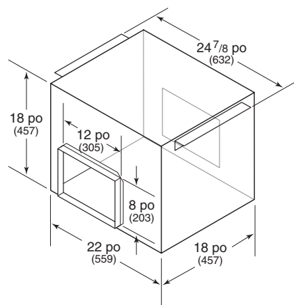
Ventilateur en ligne de 1 100 pi³/min
