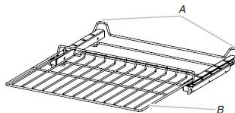
A. Rieles de deslizamiento B. Estante deslizable
