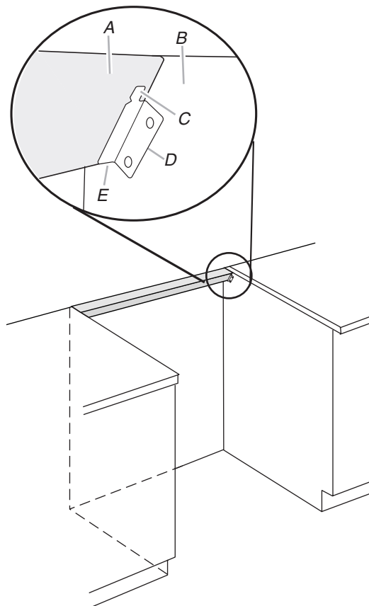
A. Planchette de remplissage B. Côté du placard C. Patte de la bride de montage D. Bride de montage E. Patte pliée de la bride de montage, pour support
