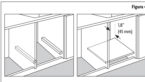
Instalación debajo de la encimera
