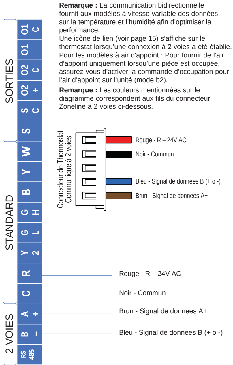
Diagramme 1 : Câblage de communication à 2 voies (5 broches / 4 fils) - utilisé avec les modèles AZV et AVV
