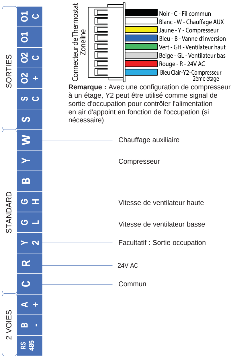
Diagramme 5 : Câblage de communication standard (chaleur : 1 / froid : 1)
