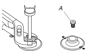
A. Propane gas orifice spud
