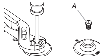
A. Injecteur à orifice pour gaz naturel
