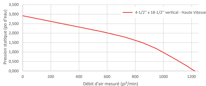
Ventilateur double
