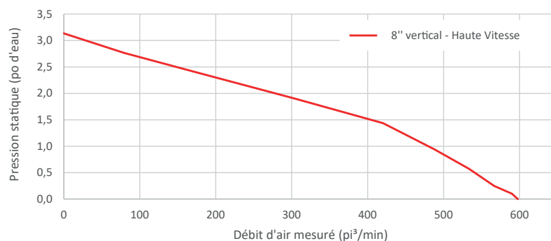
Ventilateur simple
