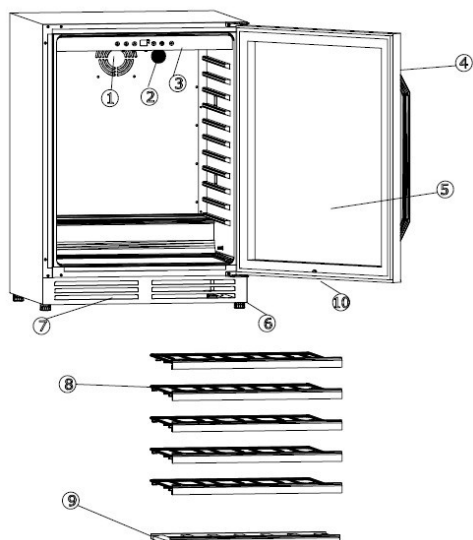
MODÈLE: WCR506SS (UNE ZONE)
