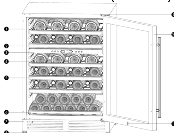
MODÈLE: WCR496DS (DEUX ZONE)
