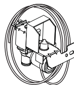
③ Ensamblaje de válvula y de tubo del agua
