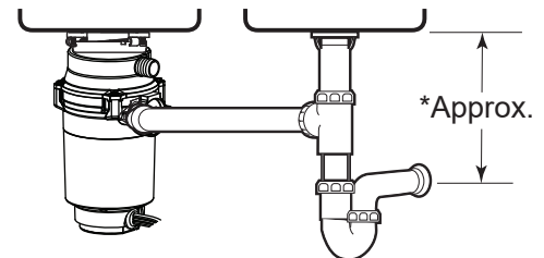
FREGADERO DOBLE CON SALIDA EN EL EXTREMO**
