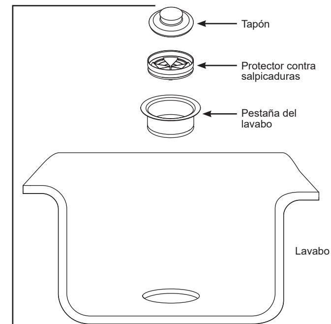
Ensamblaje del aro del fregadero
