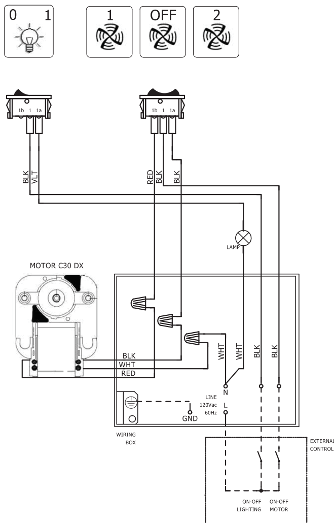
Schéma de câblage 991.0514.695
