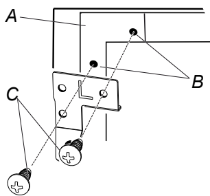
A. Taco B. Orificio piloto C. Tornillo de cabeza redonda para madera n.º 7-16 x 7/16"
