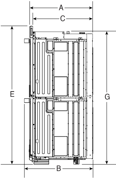
VISTA LATERAL
