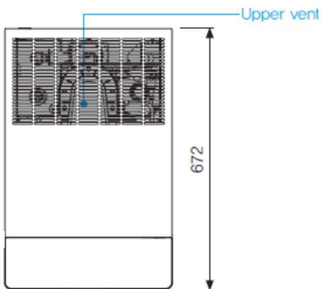
Top
