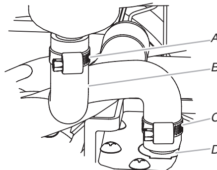
A. Bride de tuyau réglable de 7/8 po
