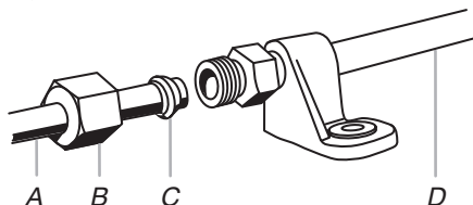
A. Línea hacia la fábrica de hielo C. Férula (se compra) B. Tuerca (adquirida) D. Línea provista de la fábrica de hielo
