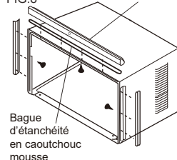
FIG.8 Rail d'angle supérieur
