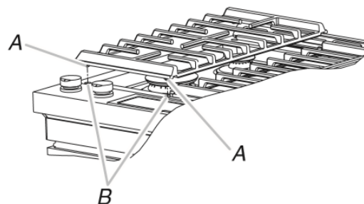
A. Butoirs B. Indentations d'alignement
