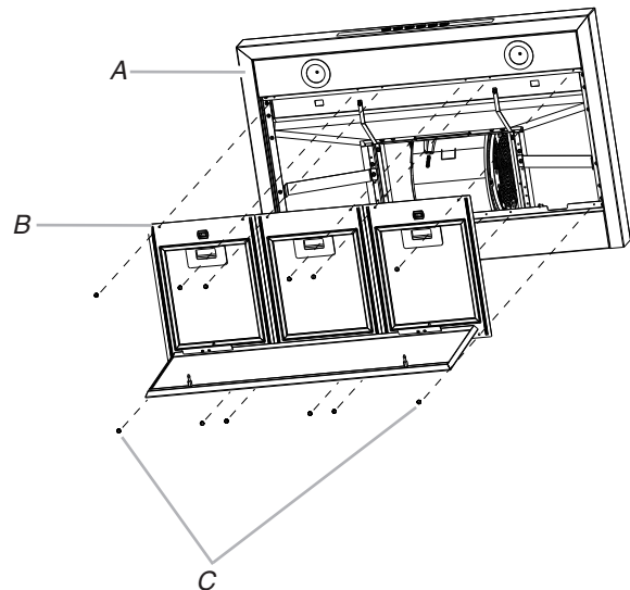
A. Hotte B. Panneau de retenue du filtre C. Vis (12)
