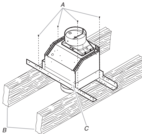
A. Vis de 5 x 45 mm (4) B. Structure solide (poteaux, solives ou traverses) C. Ventilateur déporté intelligent
