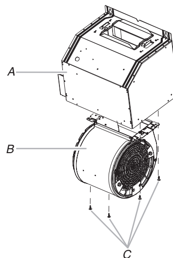
A. Caisse du ventilateur déporté B. Moteur du ventilateur C. Vis (4)
