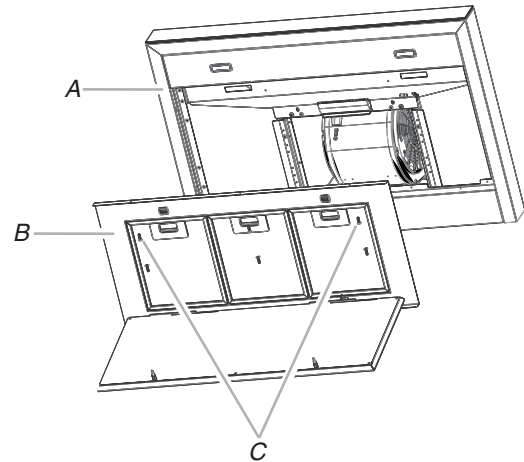
A. Hotte B. Panneau de retenue du filtre C. Vis (6)
