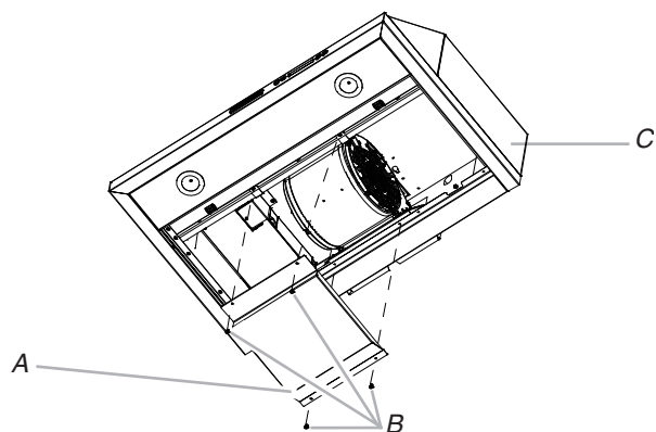
A. Couvercle du moteur du ventilateur B. Vis (4) C. Hotte
