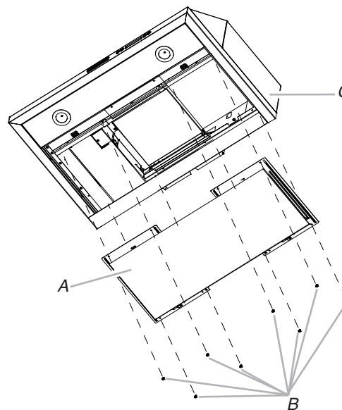
A. Bottom panel B. Screws (8) C. Range hood
