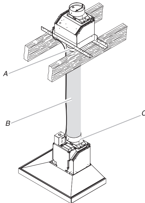
A. Raccord de transition du ventilateur déporté intelligent (en bas) B. Circuit d'évacuation C. Raccord de transition de la hotte
