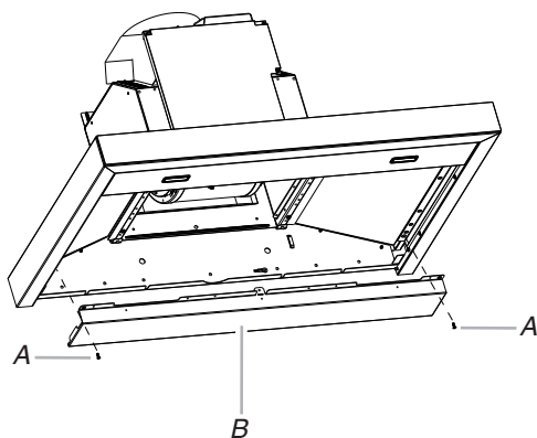
A. Vis de fixation du panneau arrière inférieur B. Panneau arrière inférieur
