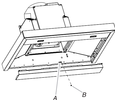
A. Capteur de température B. Vis de fixation du capteur
