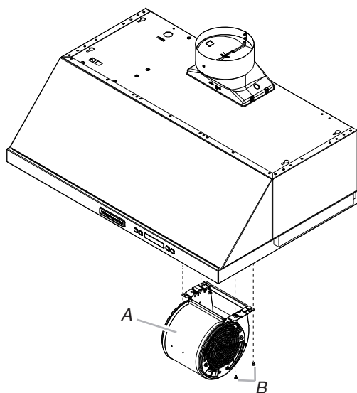
A. Moteur du ventilateur B. Vis de fixation du moteur du ventilateur (4)
