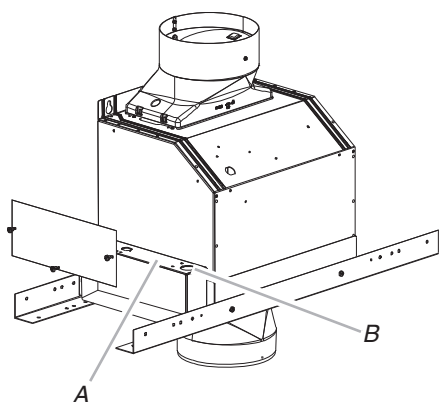
A. Boîtier de raccordement du ventilateur déporté intelligent B. Opercules arrachables
