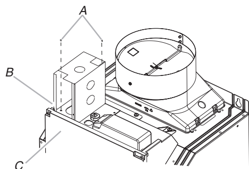
A. Vis de 3,5 x 6,5 mm (2) B. Boîtier de raccordement métallique C. Coffret électrique de la hotte
