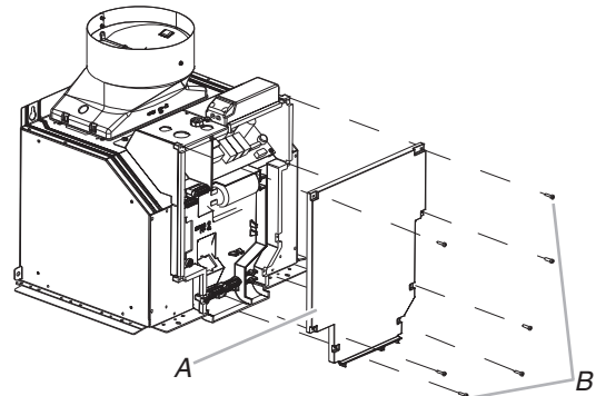
A. Couvercle en plastique du coffret électrique B. Vis (7)
