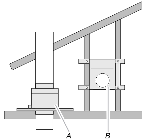
A. Montage au-dessus des solives (conduit vertical) B. Montage sur membrures fixées à une ferme (conduit horizontal)
