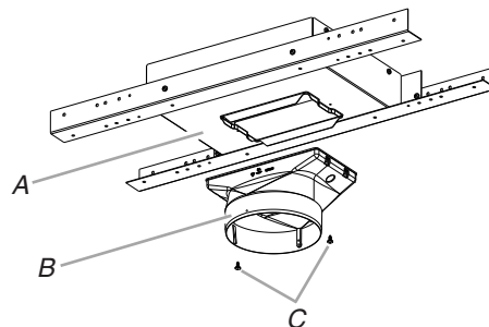
A. Base du ventilateur déporté B. Raccord de transition (sans clapet anti-reflux) C. Vis de 3,5 x 9,5 mm (2)
