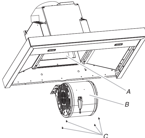
A. Caisse de la hotte B. Moteur du ventilateur C. Vis (4)
