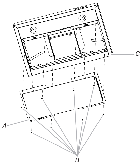
A. Bottom panel B. Screws (8) C. Range hood
