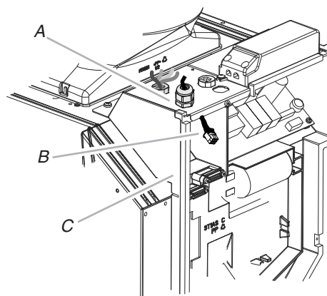
A. Serre-câble (homologation UL ou CSA) B. Connecteur de raccordement à 9 broches C. Coffret électrique de la hotte
