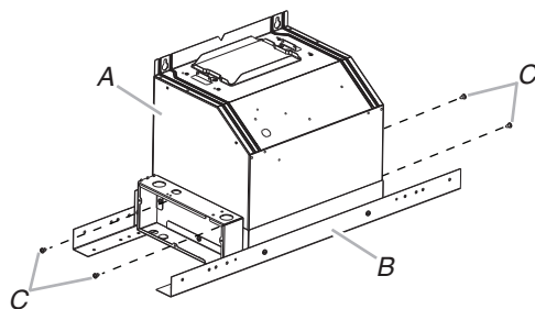
A. Caisse du ventilateur déporté B. Base du ventilateur déporté C. Vis (4)
