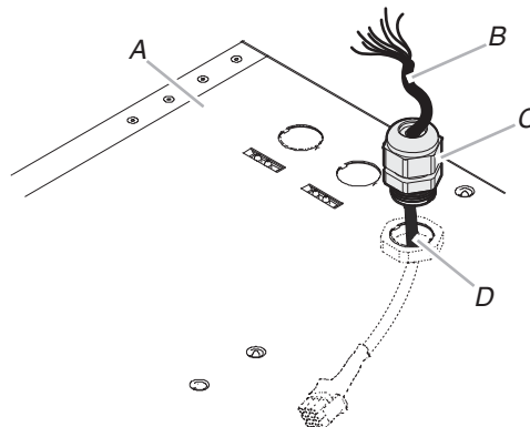
A. Hotte (haut) B. Connecteur à 9 broches (conducteurs) C. Serre-câble plastique (homologation UL ou CSA) D. Opercule arrachable
