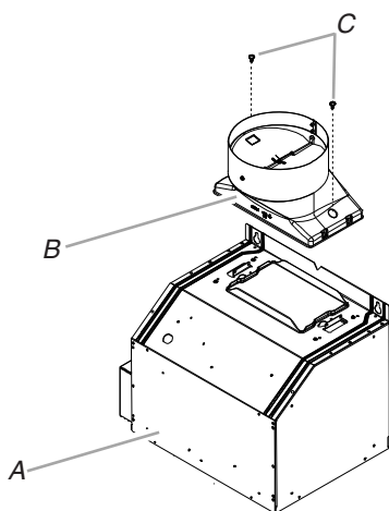
A. Caisse du ventilateur déporté B. Raccord de transition (avec clapet anti-reflux) C. Vis de 3,5 x 9,5 mm (2)
