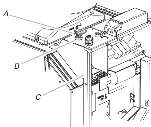
A. Conducteurs d'alimentation (4) B. Serre-fils (homologation UL ou CSA) C. Coffret électrique de la hotte
