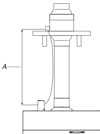
A. Distance entre le ventilateur déporté intelligent et le boîtier de raccordement de la hotte
