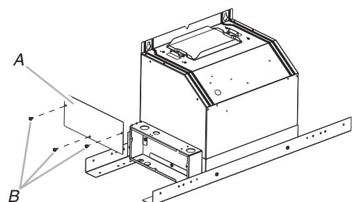
A. Couvercle du boîtier de raccordement B. Vis (3)
