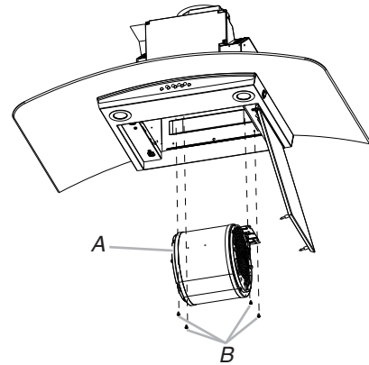
A. Moteur du ventilateur B. Vis, rondelles en acier et rondelles en caoutchouc (4)
