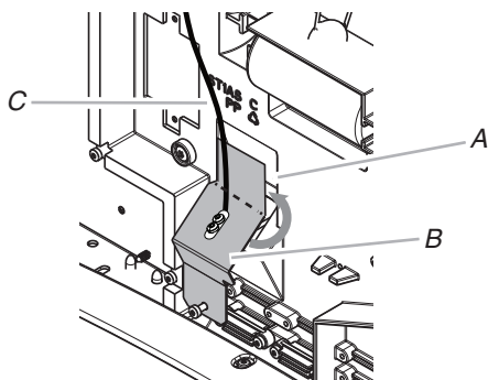
A. Ouverture B. Couvercle C. Conducteur de terre du couvercle
