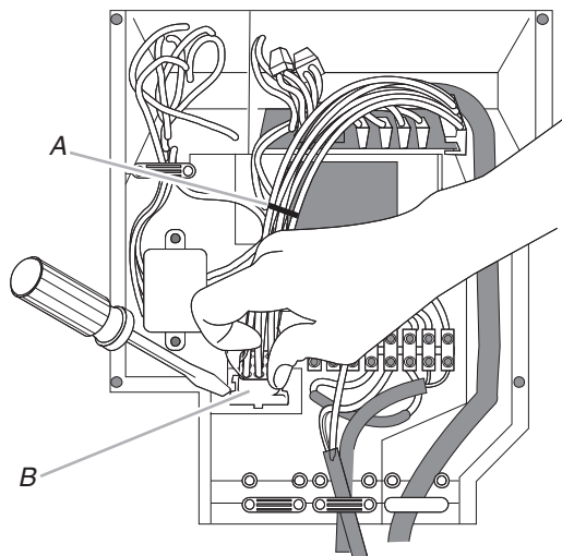
A. Attache-câble B. Connecteur à 9 broches (conducteurs)
