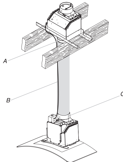
A. Raccord de transition du ventilateur déporté intelligent (en bas) B. Circuit d'évacuation C. Raccord de transition de la hotte
