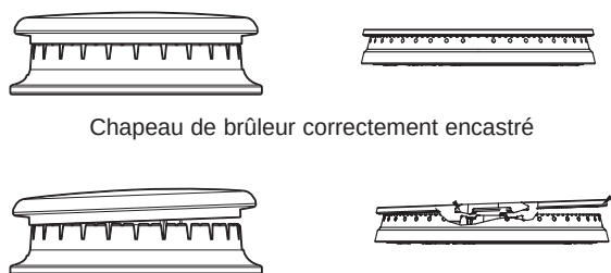
Chapeau de brûleur incorrectement installé
