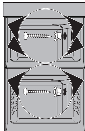
Figure 7: Ubicaciones de los tornillos antivuelco
