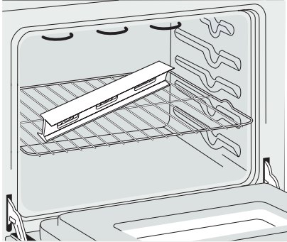
Figure 8: Nivelación
