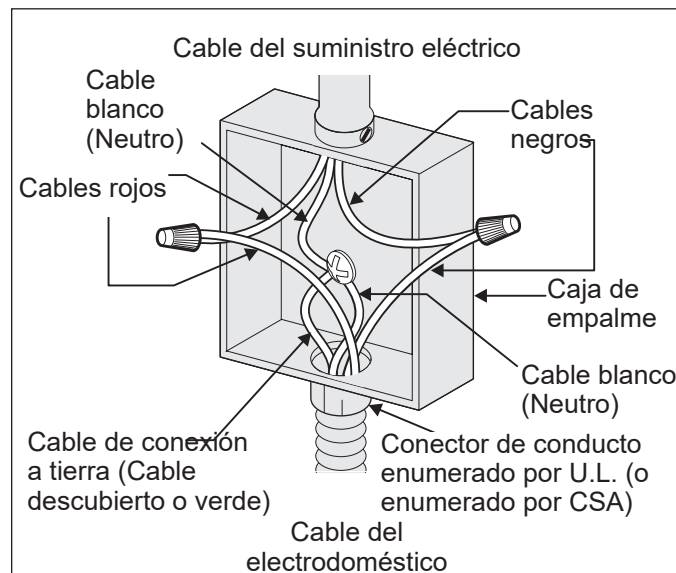
Figure 3: Caja de empalme de conexión a tierra de 3 cables
