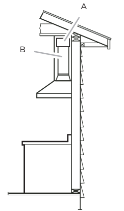
A. Déflecteur B. Conduit rond de 6" (15,2 cm)
