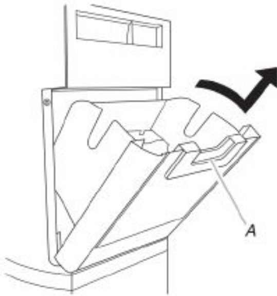
A. Levier de dégagement
