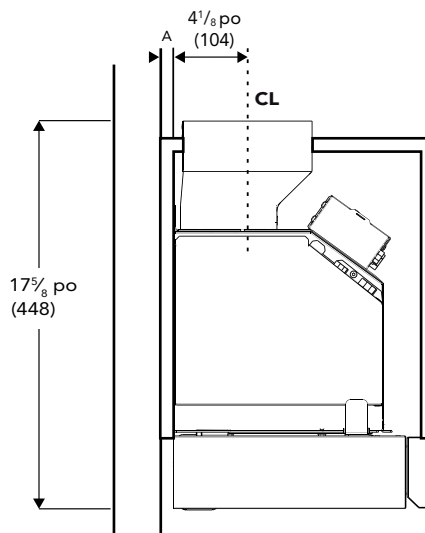
A. Épaisseur de la matière du mur arrière de l'armoire
