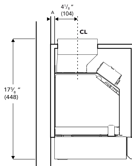
A. Espesor del material de la pared posterior del gabinete
