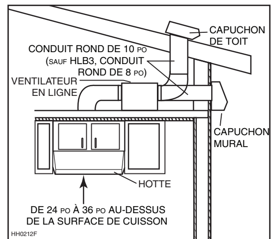
INSTALLATION TYPE AVEC VENTILATEUR EN LIGNE MODÈLE ILB3, ILB6, ILB9 OU ILB11
