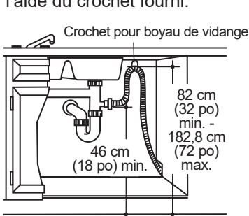
Installation avec raccord en T
