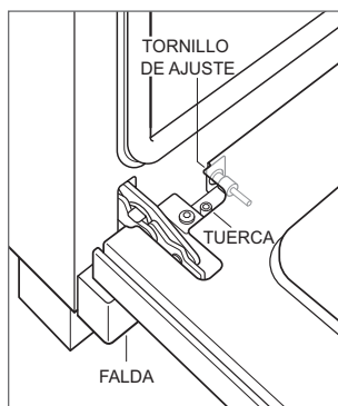
Alineamiento de la puerta
