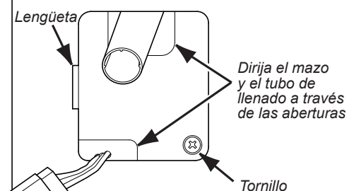
Reinstalación de la cubierta plana
