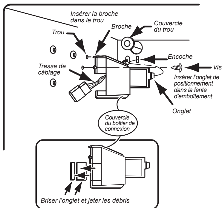
Couvercle du logement du câblage de la machine à glaçons
