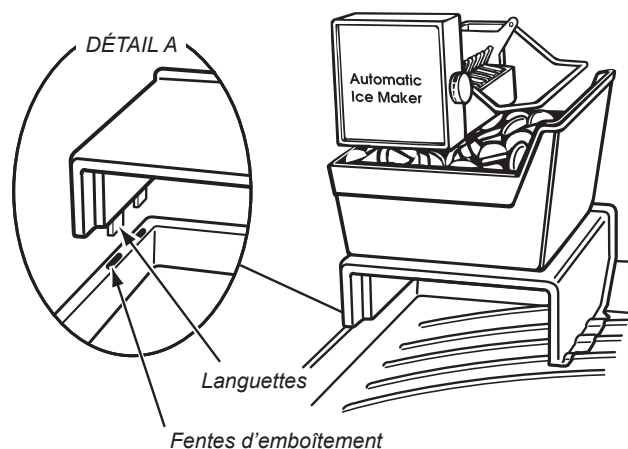
Fentes d'emboîtement
