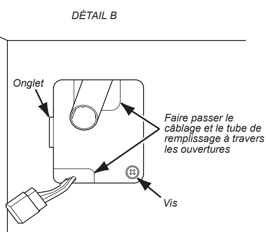
Réinstallation du couvercle plat
