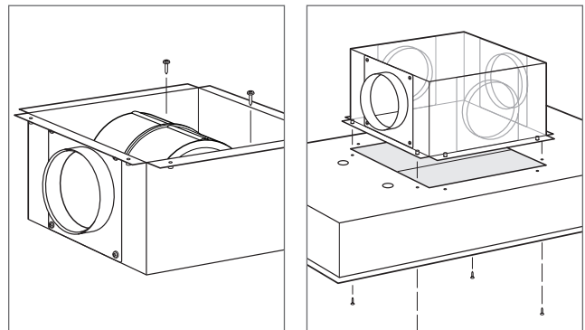
Instalación del extractor interno Dirección de la descarga
