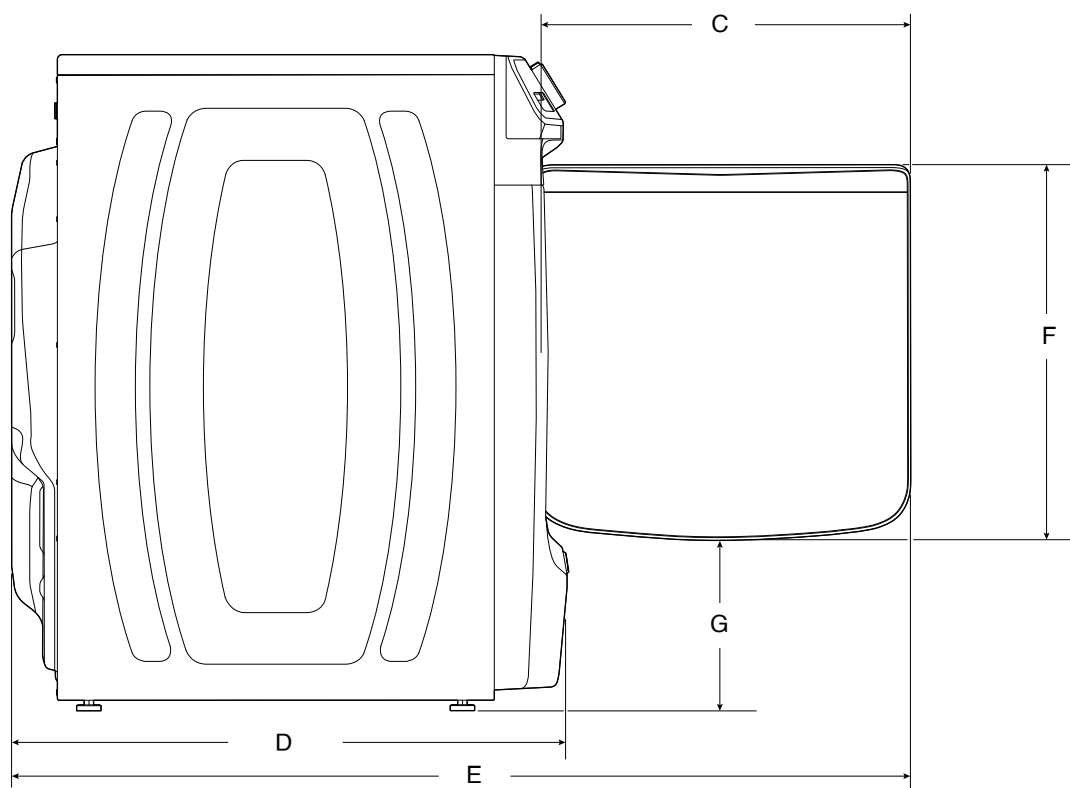
VUE LATÉRALE
