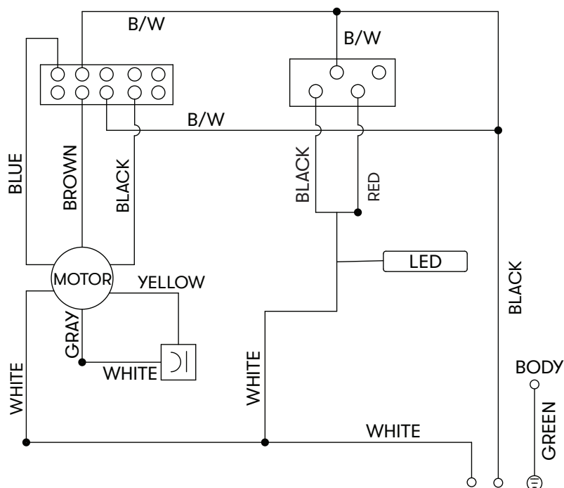
AK1124Bx Wiring Diagram
