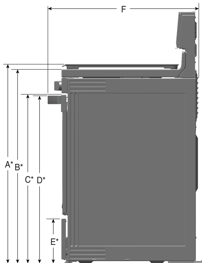
VUE LATÉRALE
