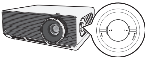
Dial de ajuste de la posición de la pantalla de proyección (lente)
