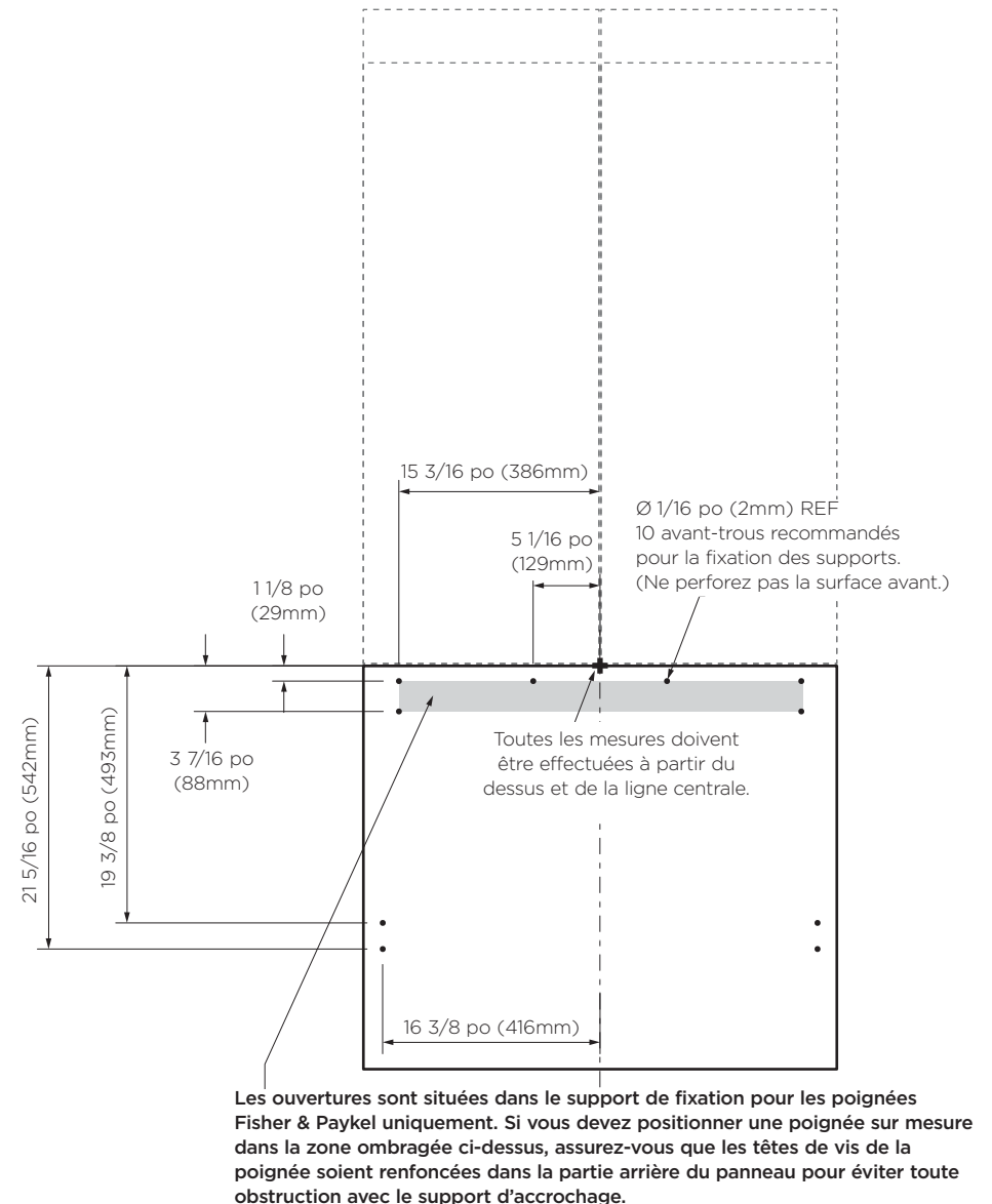
PANNEAU INFÉRIEUR — VUE ARRIÈRE
