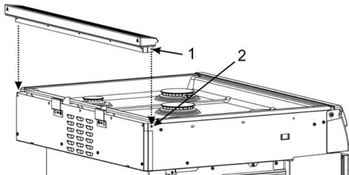
Figure 2: Colocación de la moldura para islas
