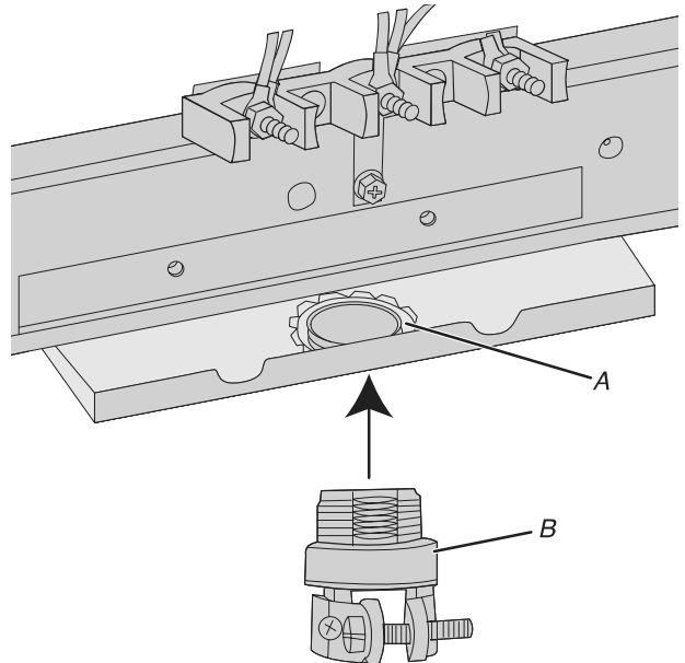
A. Tuerca de retención removible
