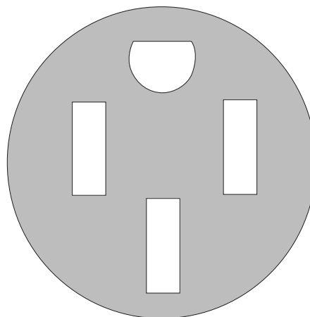
Prise murale à 4 fils (14-50R)
