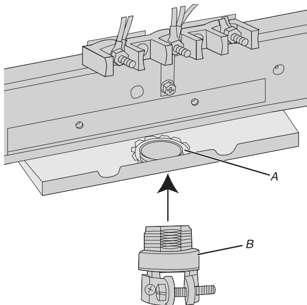
A. Écrou de retenue amovible
