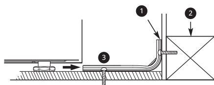
1 Soporte antivuelco
