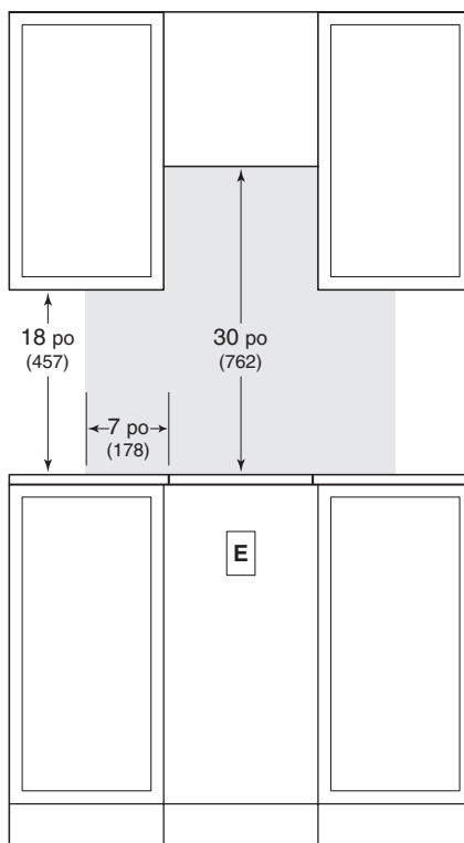
VUE AVANT
